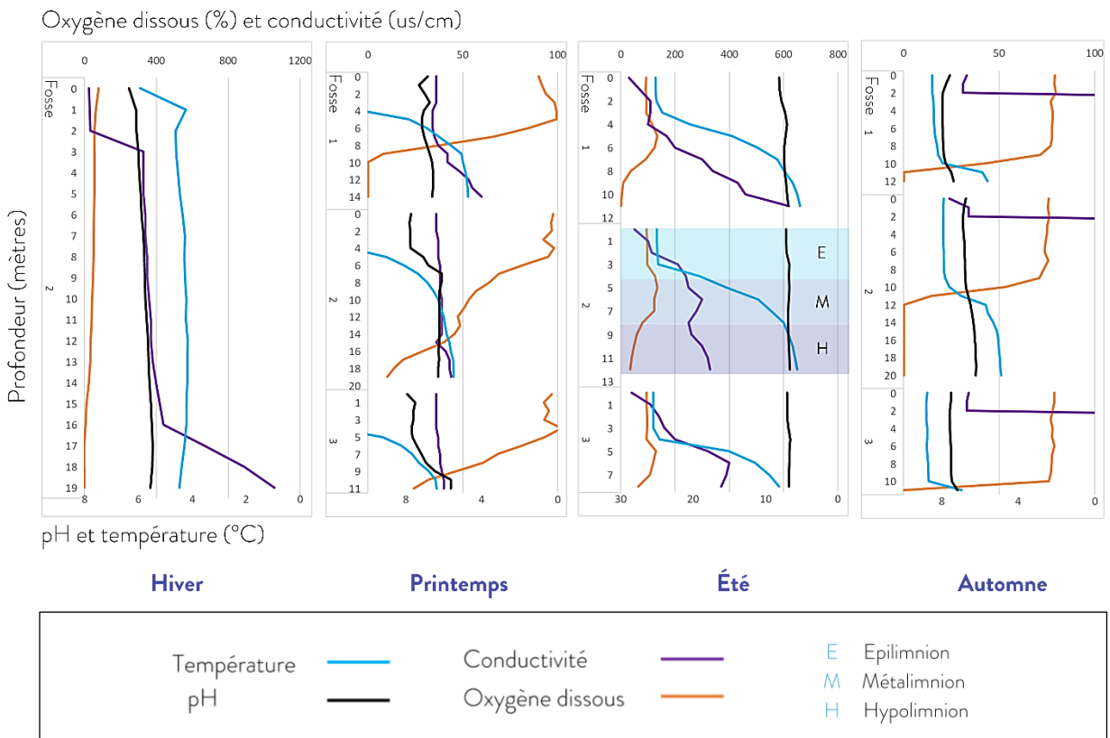
Figure 6 : Profils physico-chimiques du lac Thomas, 2023-2024
